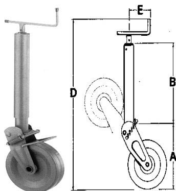
Stützräder mit halbautomatischem Klappvorgang und Federverriegelung
