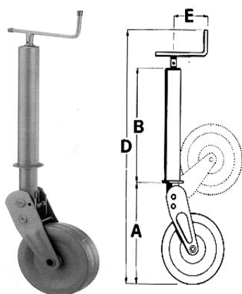
Stützräder mit vollautomatischer Klapp-Verriegelung
