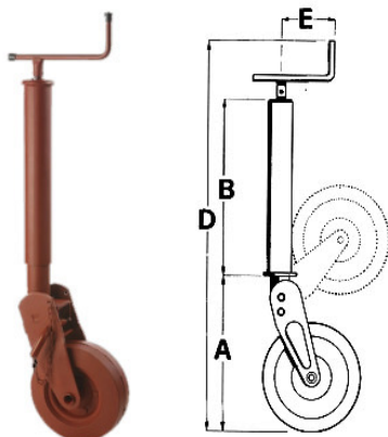
Stützräder von Hand zu klappen
